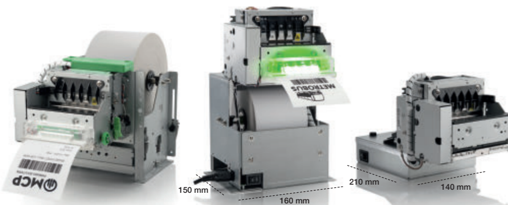
Guide de sortie clignotant à DEL programmable sur la TUP500
